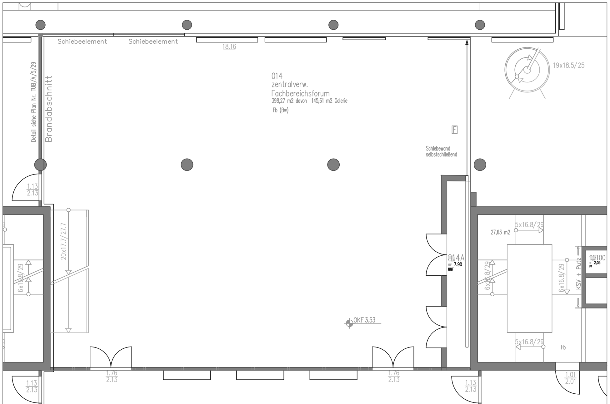
Erdgeschoss
